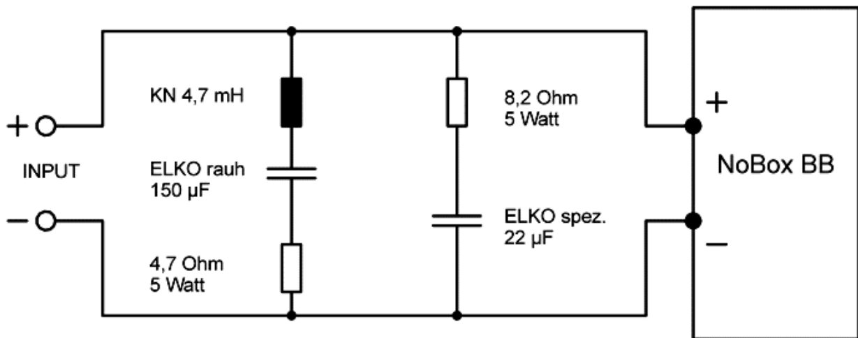
Impedanzlinearisierung NoBox BB - Stand 03.06.2004
